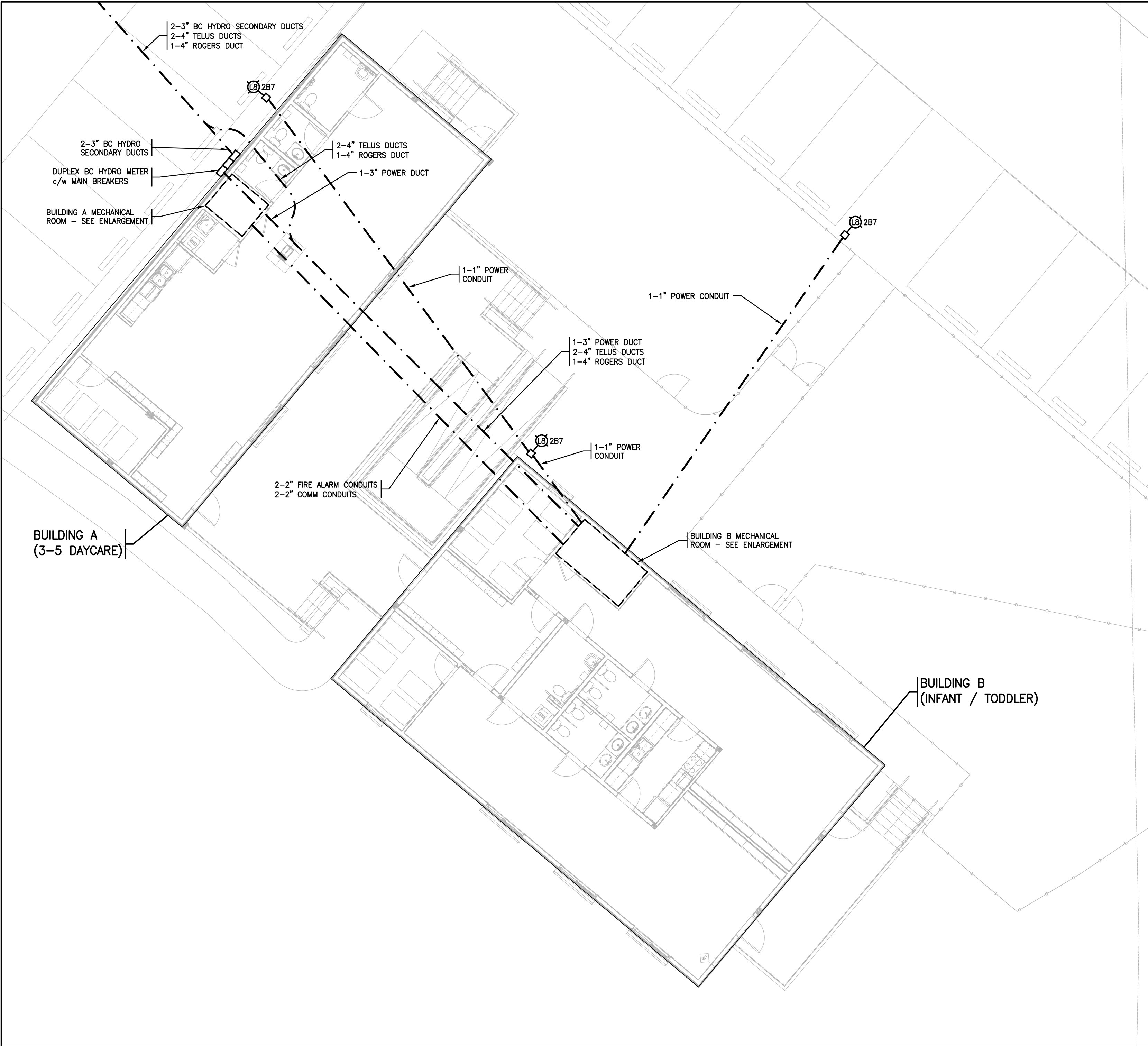
A SITE PLAN ENLARGEMENT SCALE: 1:100
