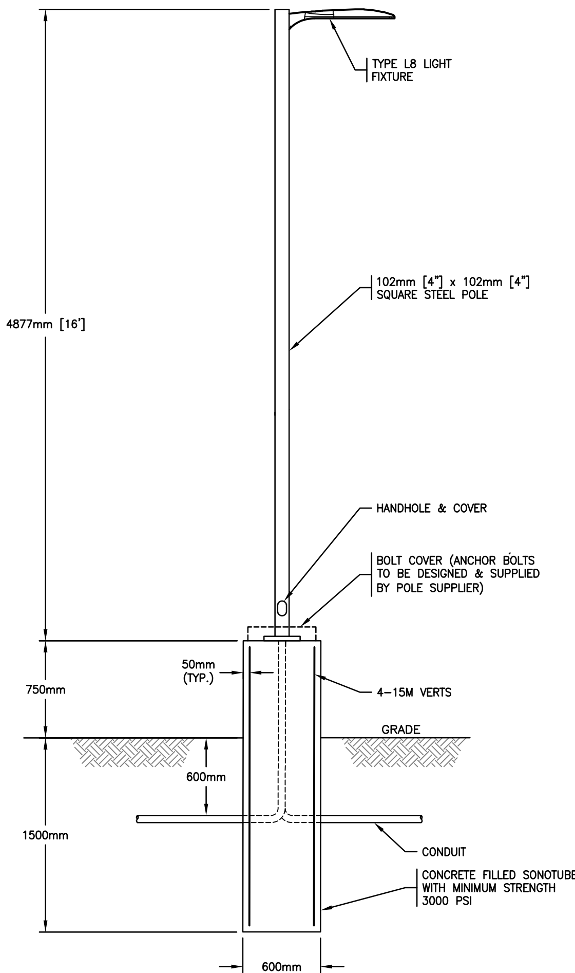
PARKING LOT LUMINAIRE (TYPE L8) SCALE: N.T.S.
